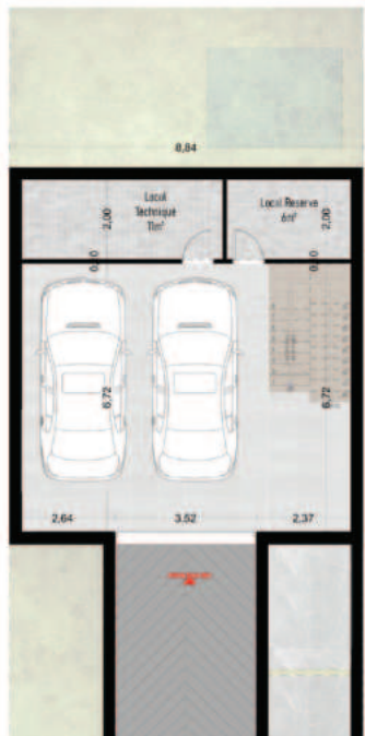
Plan sous-sol
